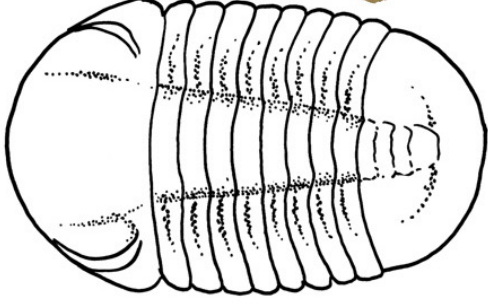
Trilobiten Symphysurus hade inga utstickande delar. Man har funnit fossil efter den i Västergötland och på Öland.
