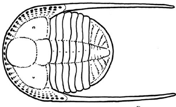
Trilobiten Tretaspis hade långa bakåtgående spröt på sin huvudsköld, men dessa finns sällan kvar i fossilen. Tretaspis har hittats i Västergötland.
